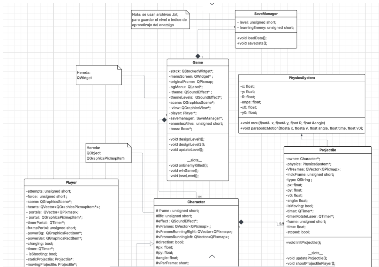
Figura 1: Diagrama de clases parte I (Archivo adjunto en el repositorio)
